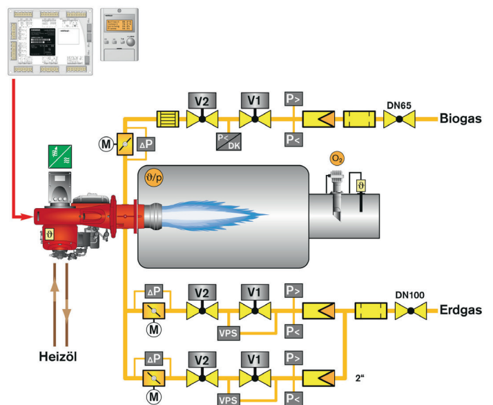
W-FM200 Beispiel für Zweigasbrenner und Simultanbetrieb mit einem W-FM200 Feuerungsmanager.
