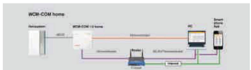
Funktionsumfang der Kommunikationsmodule WCM-COM expert und WCM-COM home.
