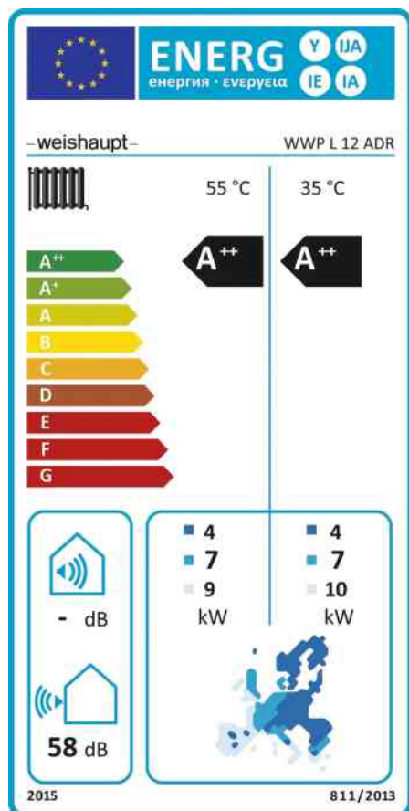
ErP-Label für eine Luft/Wasser-Wärmepumpe.
