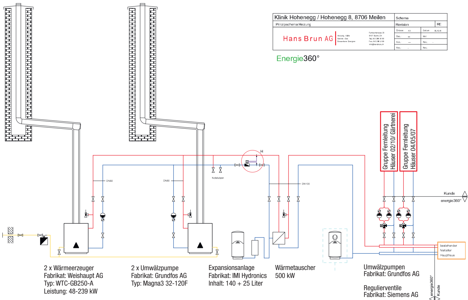
Schema der Anlage in der Hohenegg. Links die beiden WTC GB 250, in der Mitte die Systemtrennung durch einen Wärmetauscher.
