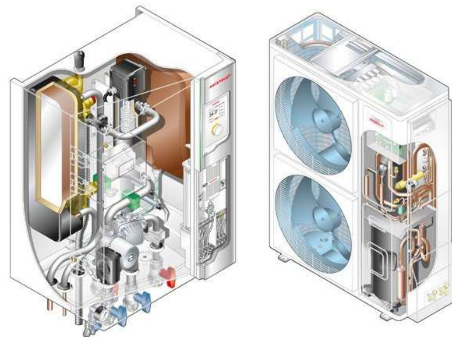
Hydraulikeinheit der neuen Split- wärmepumpe
