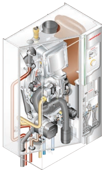
Schnittbild des neuen Gas-Brennwertgeräts WTC-GW 15/25-B.
