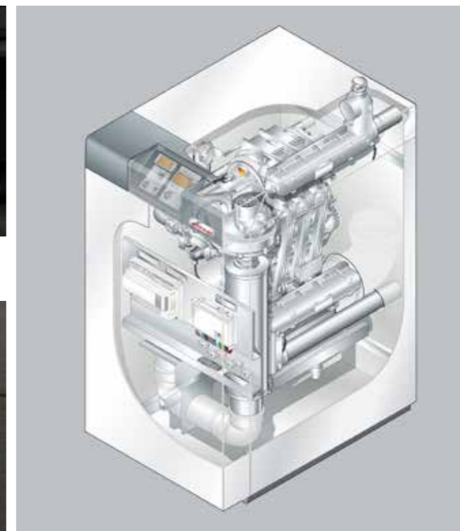
Schnittzeichnung eines Weishaupt-Brennwertkessels.
