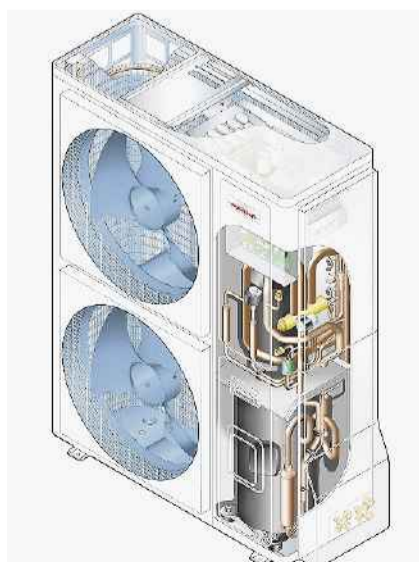
Schnittgrafik des Aussengerätes der neuen Splitwärmepumpe.
